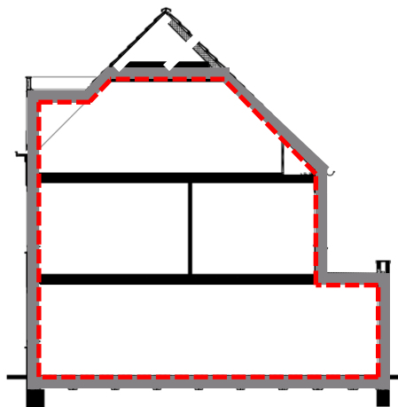
Figuur 2b: Te meten zone valt binnen de thermische schil (= luchtdichte schil); de vliering ligt buiten de thermische schil; vlizoluiken/knieschotten behoren tijdens de meting gesloten te zijn – zie hiervoor paragraaf 5.1.5.
