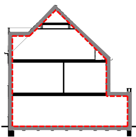
Figuur 2a: Te meten zone valt binnen de thermische schil (= luchtdichte schil); ook de vloering ligt binnen de thermische schil; vliedolijken behoren tijdens de meting open te zijn; knieschotten behoren tijdens de meting gesloten te zijn – zie hiervoor paragraaf 5.1.5.
