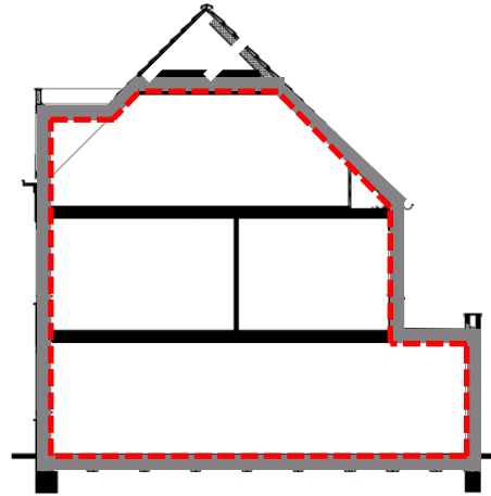
Figuur 2b: Te meten zone valt binnen de thermische schil (= luchtdichte schil); de vloering ligt buiten de thermische schil; vliedolijken/knieschotten behoren tijdens de meting gesloten te zijn – zie hiervoor paragraaf 5.1.5.
